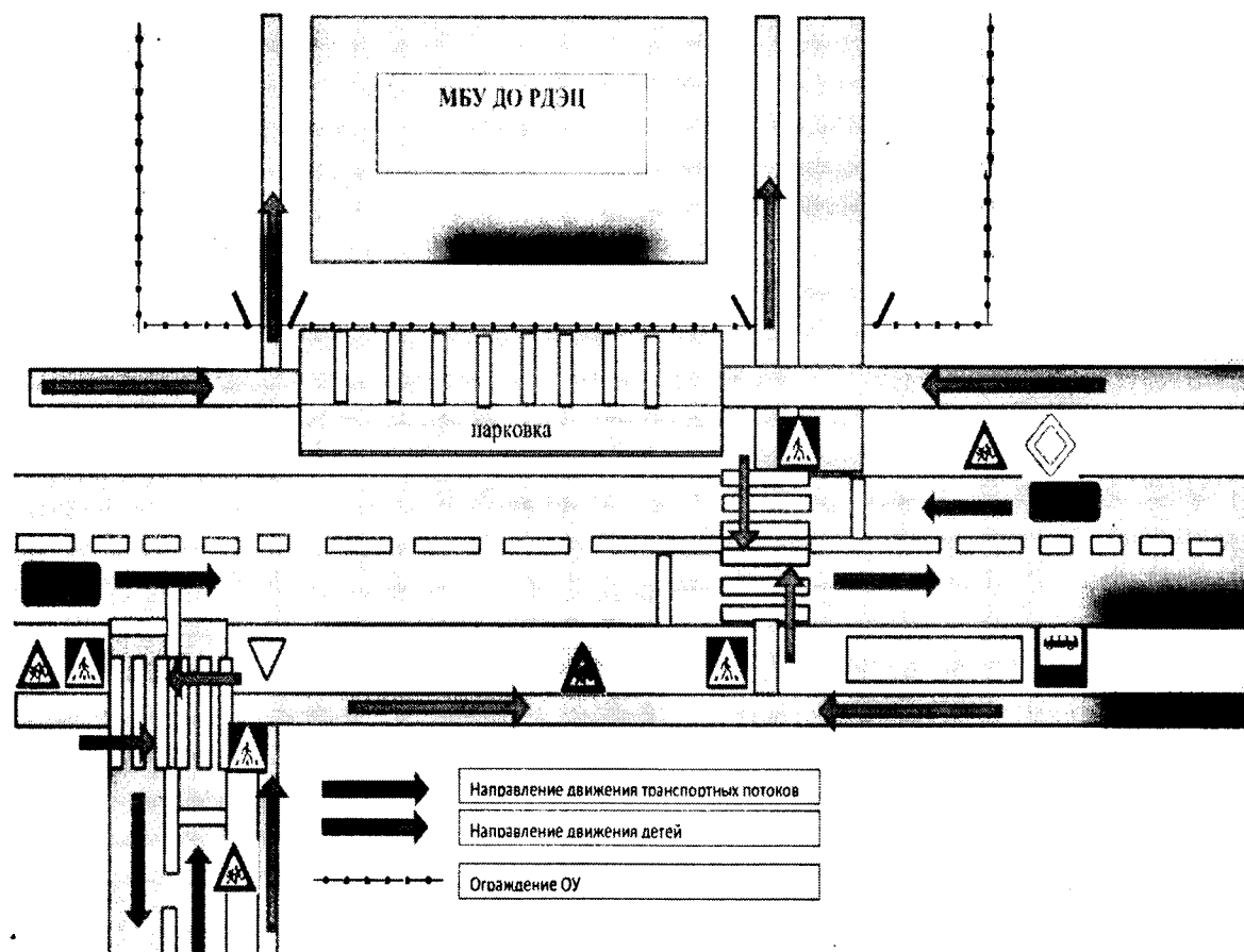
2. Схема организации дорожного движения в непосредственной близости от МБУ ДО РДЭЦ, с размещением соответствующих технических средств организации дорожного движения, маршрутов движения детей и расположения парковочных мест
